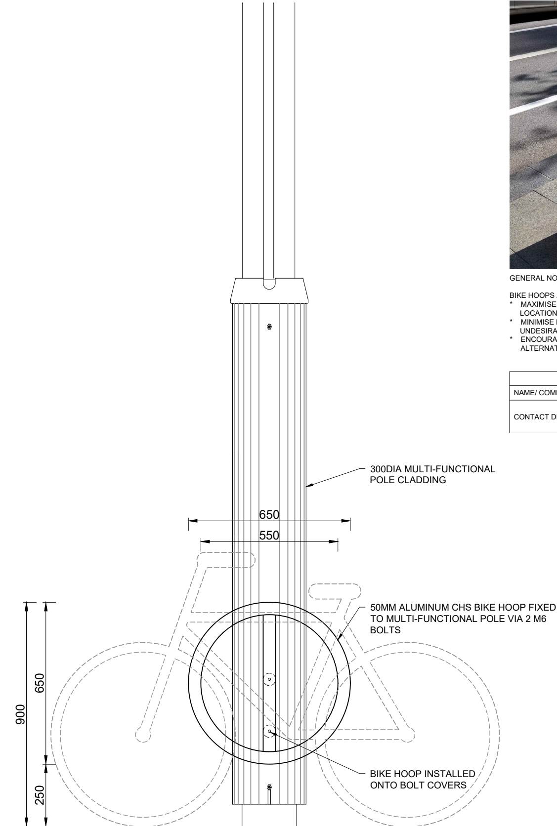
ELEVATION
