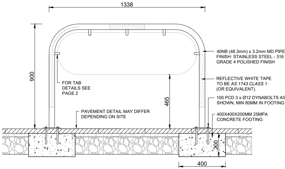
B ELEVATION
