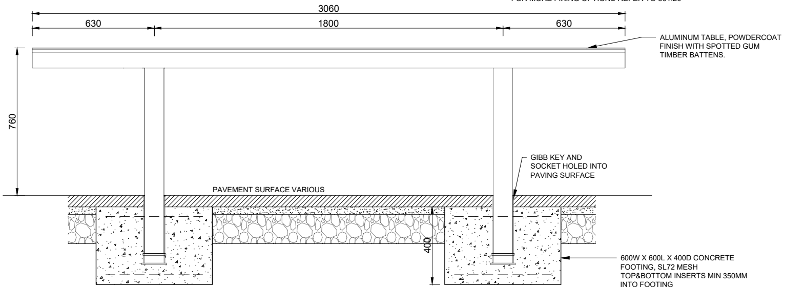
(B) SIDE ELEVATION - TABLE
